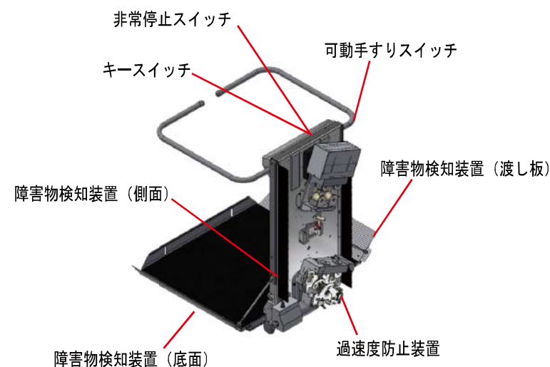
非常停止スイッチ 緊急時に非常停止スイッチを押すと即座に動作が停止します。スイッチを開放すると簡単に復旧します。
